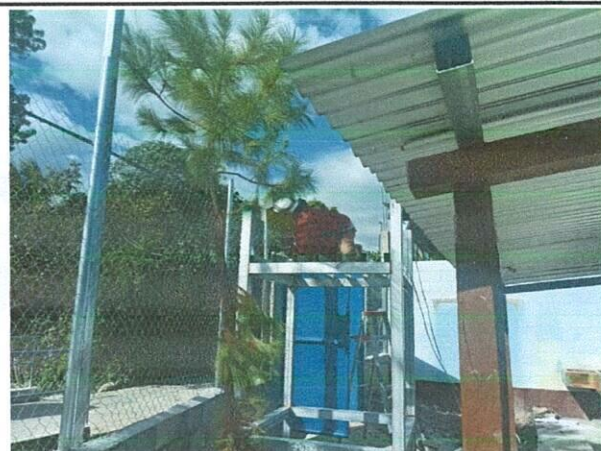
Foto 3: Área en la que se está llevando a cabo el mejoramiento e instalación de un tanque elevado destinado al almacenamiento de agua.
